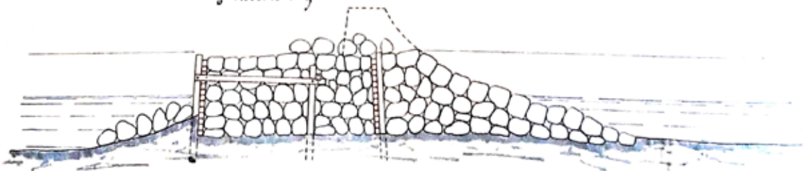
Sektion e-f
