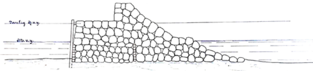
Sektion a-b
